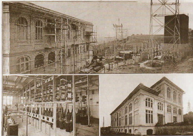
ESTACIÓN CENTRAL TRANSFORMADORA DE SAN (110.000 VOLTS)
